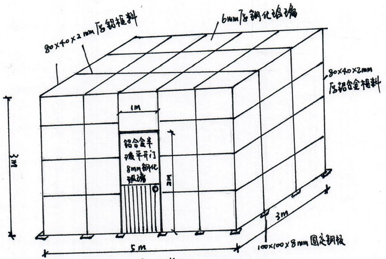
阳光房大样
