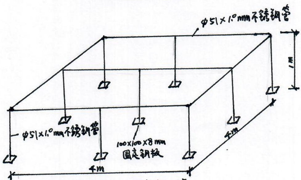
不锈钢晒衣架大样
